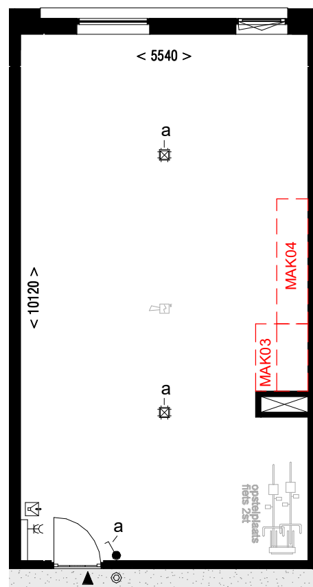
Derde verdieping, 11650+P
