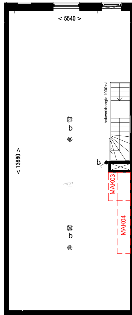
Eerste verdieping, +4850 Peil
