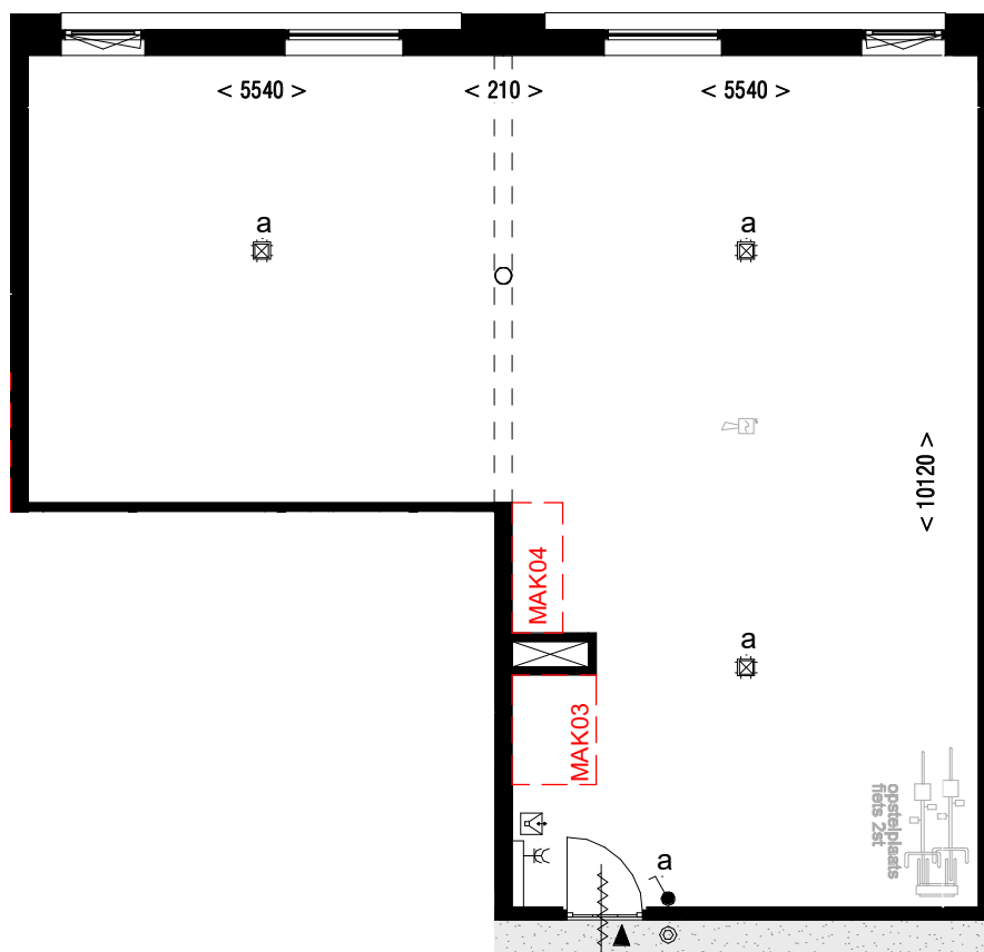
Tweede verdieping, 8250+P
