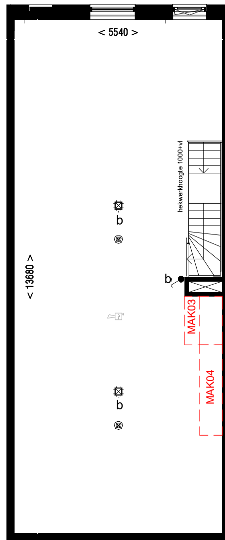
Eerste verdieping, +4850 Peil
