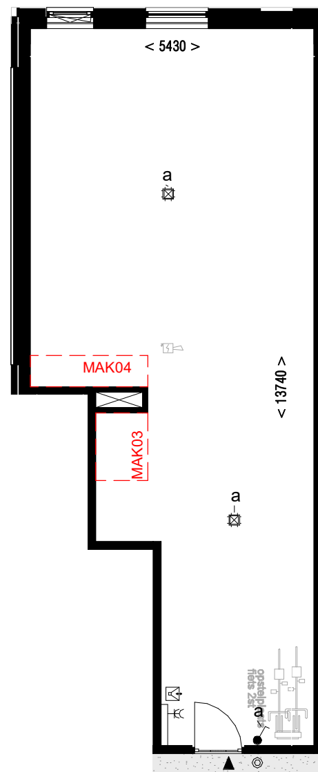
Tweede verdieping, 8250+P
